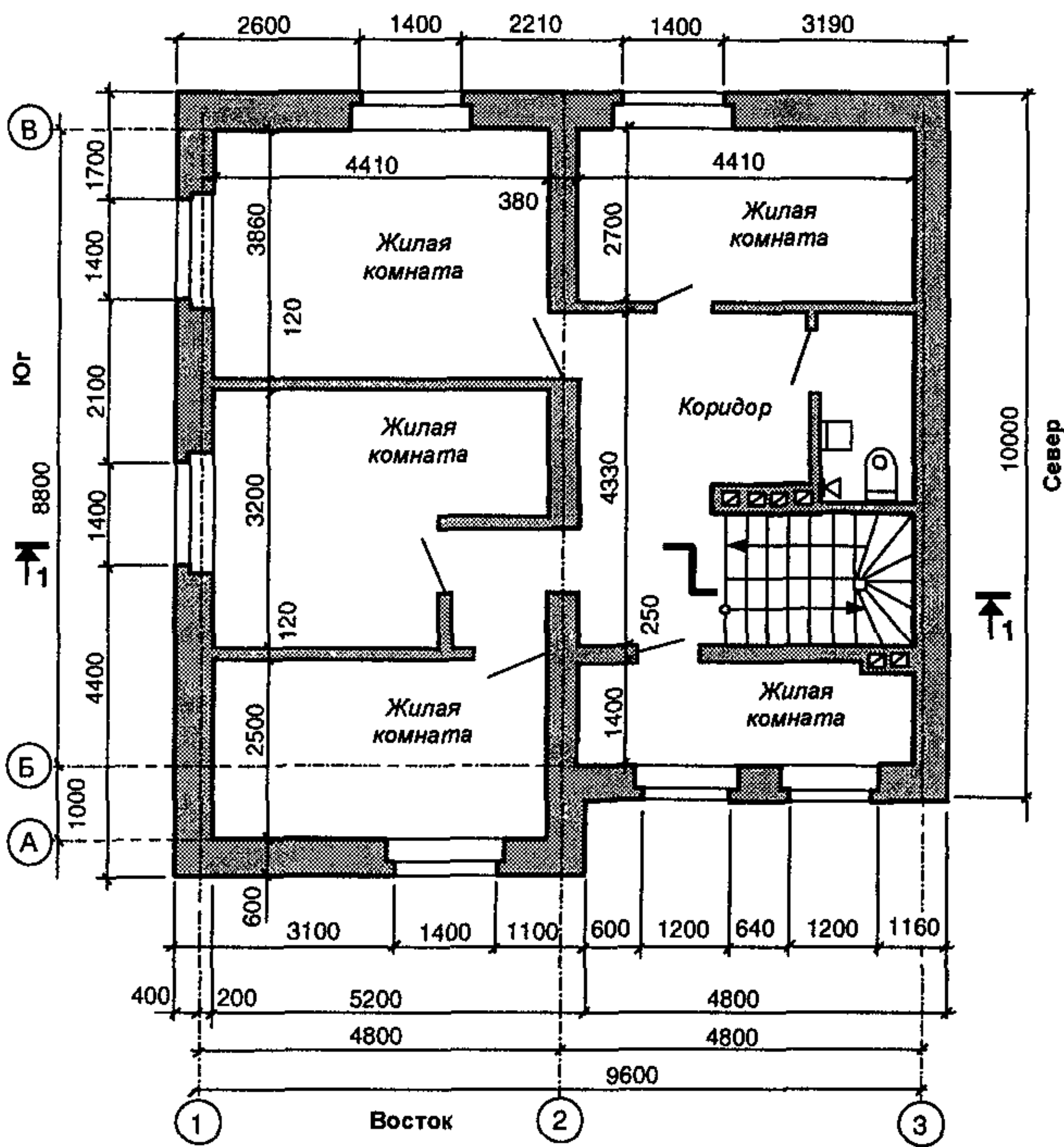
План 1-го этажа
